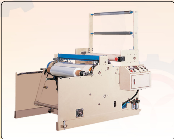
TYPE : TE2 (Auto. cut & auto. change reel, back cutter type) 自動切割&自動換捲，後飛刀型式
