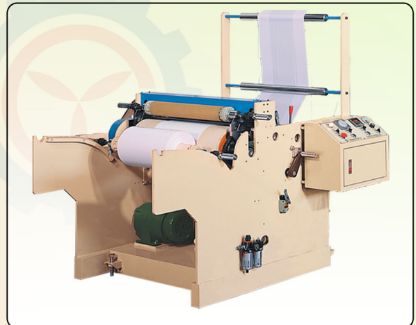
TYPE : H2 (Auto. cut & manual change reel) 自動切割&手動換捲
