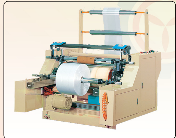
TYPE : T2 (Auto. cut & auto. change reel, front cutter type) 自動切割&自動換捲，前飛刀型式
