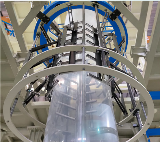
4-D Motorized Guiding Cage 4-D 電動安定環
