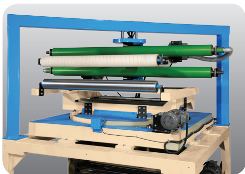
360° Oscillating Nip Roller Device (Horizontal Type) 360° 上旋轉（水平式）
