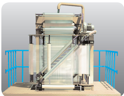
360° Oscillating Nip Roller Device (Vertical Type) 360° 上旋轉（垂直式）
